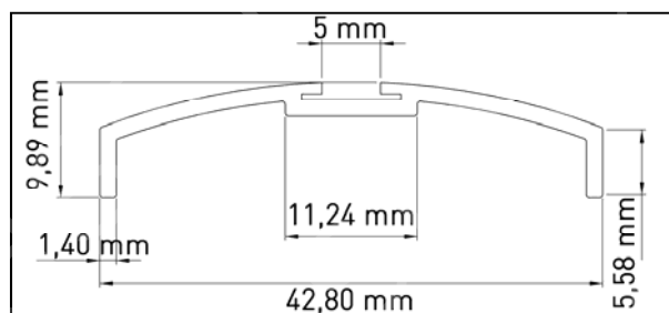
Copre - binario
