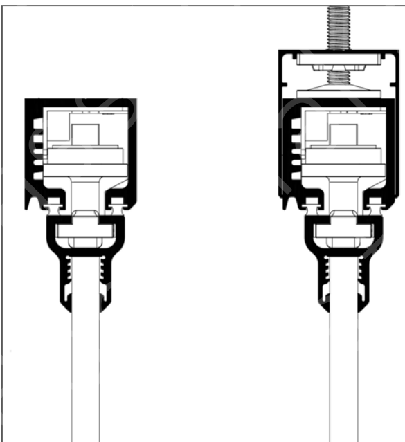
Profili superiori
