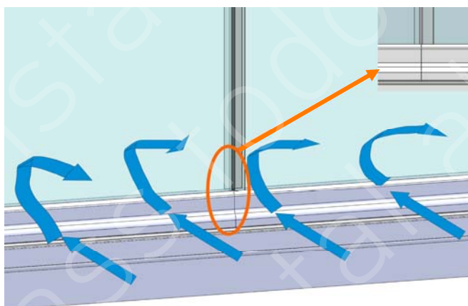
Sistema Todocrystal
