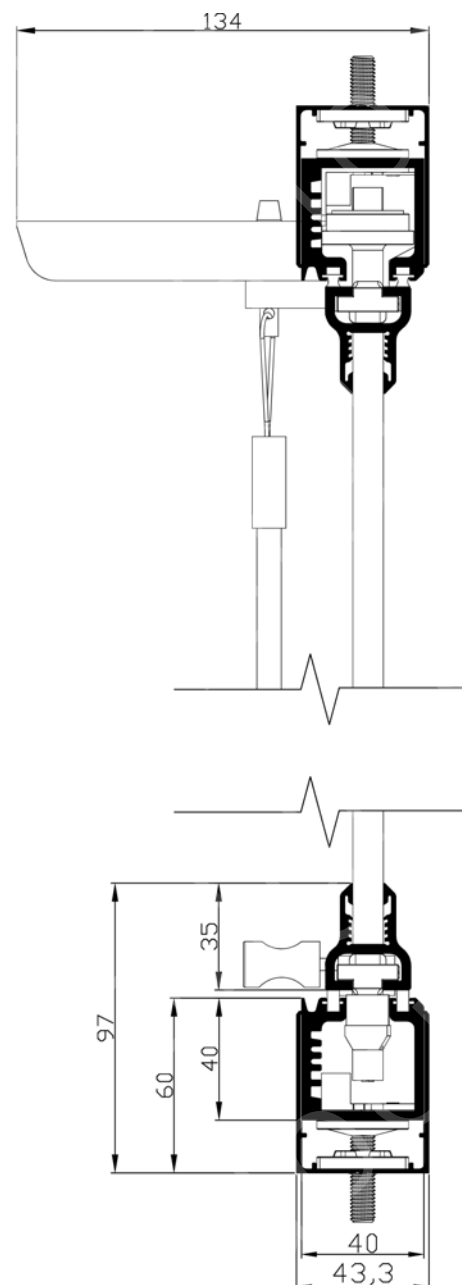
Sezioni verticali, con compensatore superiore e inferiore
