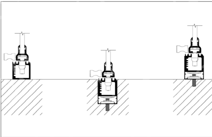
Profili inferiori
